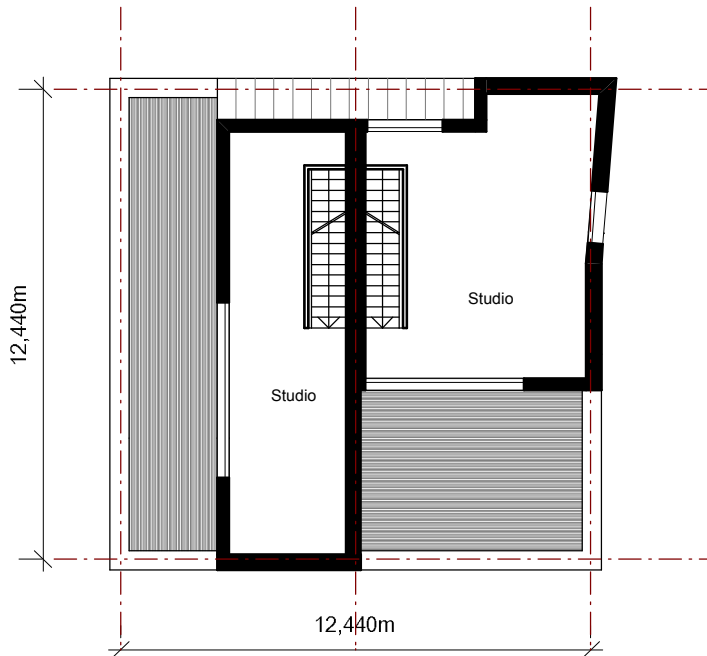
DG_Typ Doppelhaus ( 2/3 Geschoss )
